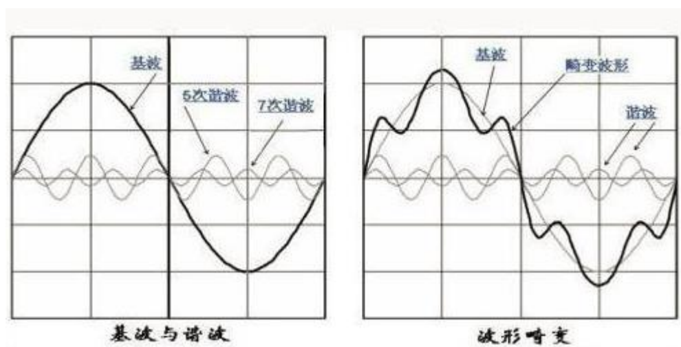
图 1 谐波图
