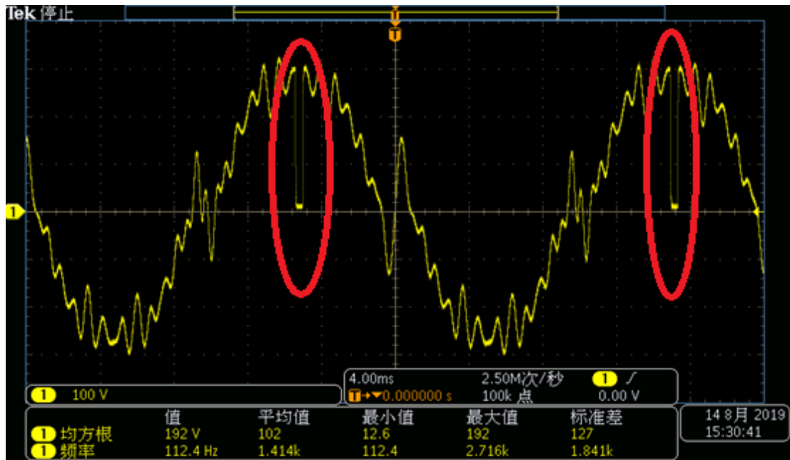
图 5 IT-M7700 谐波模拟示波器图
